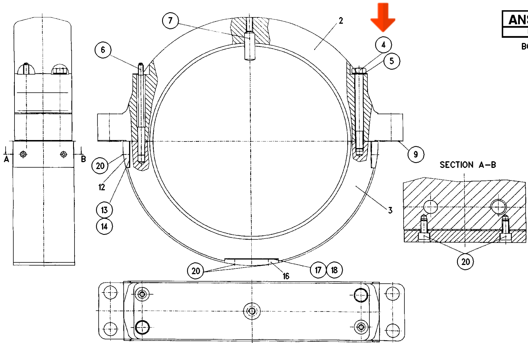
ANELLO ALLOGGIAMENTO CUSCINETTO ADJUST RING
