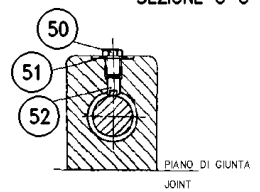
SECTION C-C SEZIONE C-C
