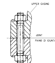
SECTION D-D SEZIONE D-D
