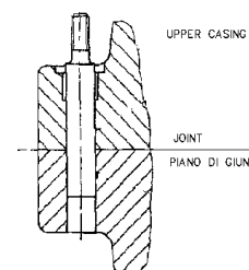
SECTION D-D SEZIONE D-D
