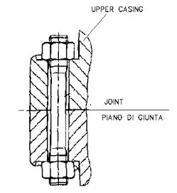
SECTION D-D SEZIONE D-D
