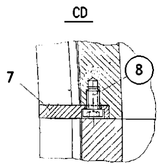
MONTAGGIO DELLE PARTI INTERNE ASSEMBLY OF INTERNALS
