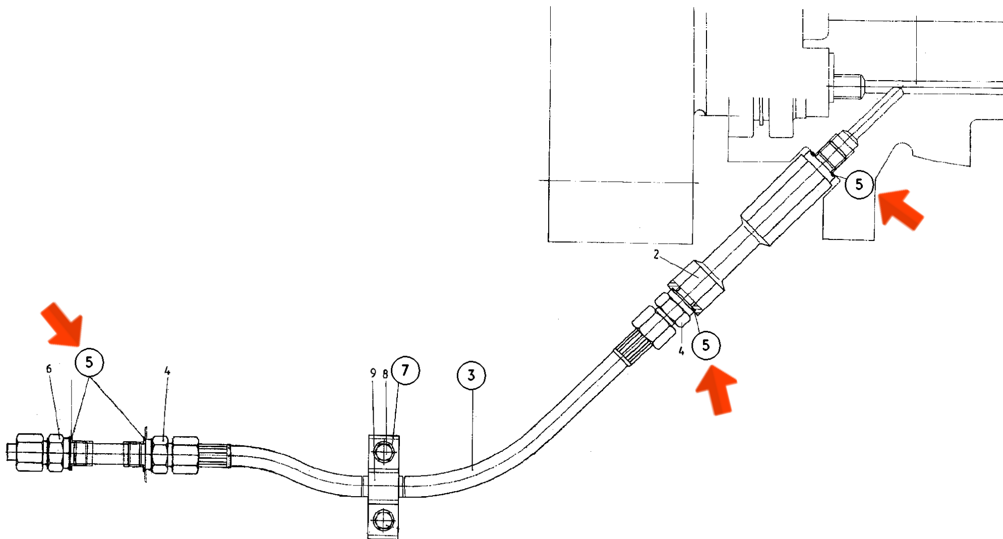
SISTEMA OLIO SOLLEVAMENTO CUSCINETTO ROTORE COMPR. COMPRESSOR BEARING LIFTING OIL SYSTEM
