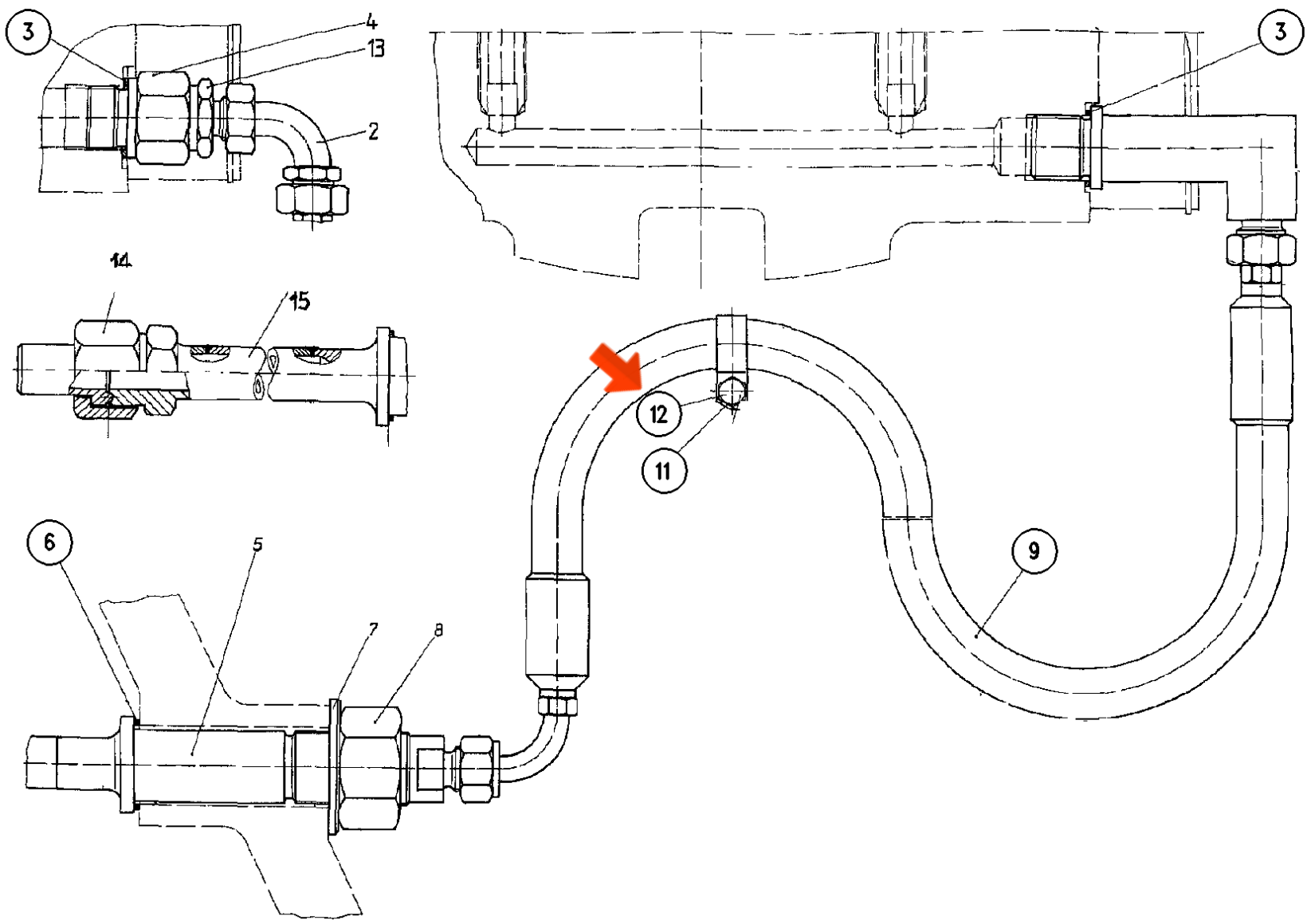
SISTEMA OLIO SOLLEVAMENTO ROTORE CUSCINETTO TURBINA TURBINE BEARING LIFTING OIL SYSTEM
