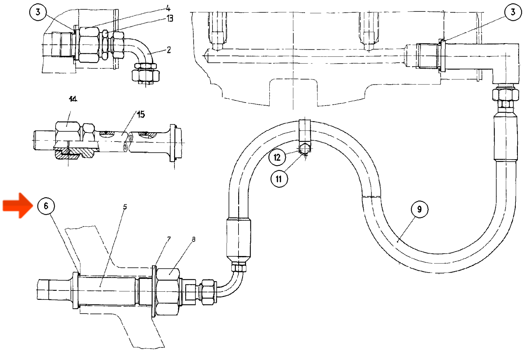
SISTEMA OLIO SOLLEVAMENTO ROTORE CUSCINETTO TURBINA TURBINE BEARING LIFTING OIL SYSTEM
