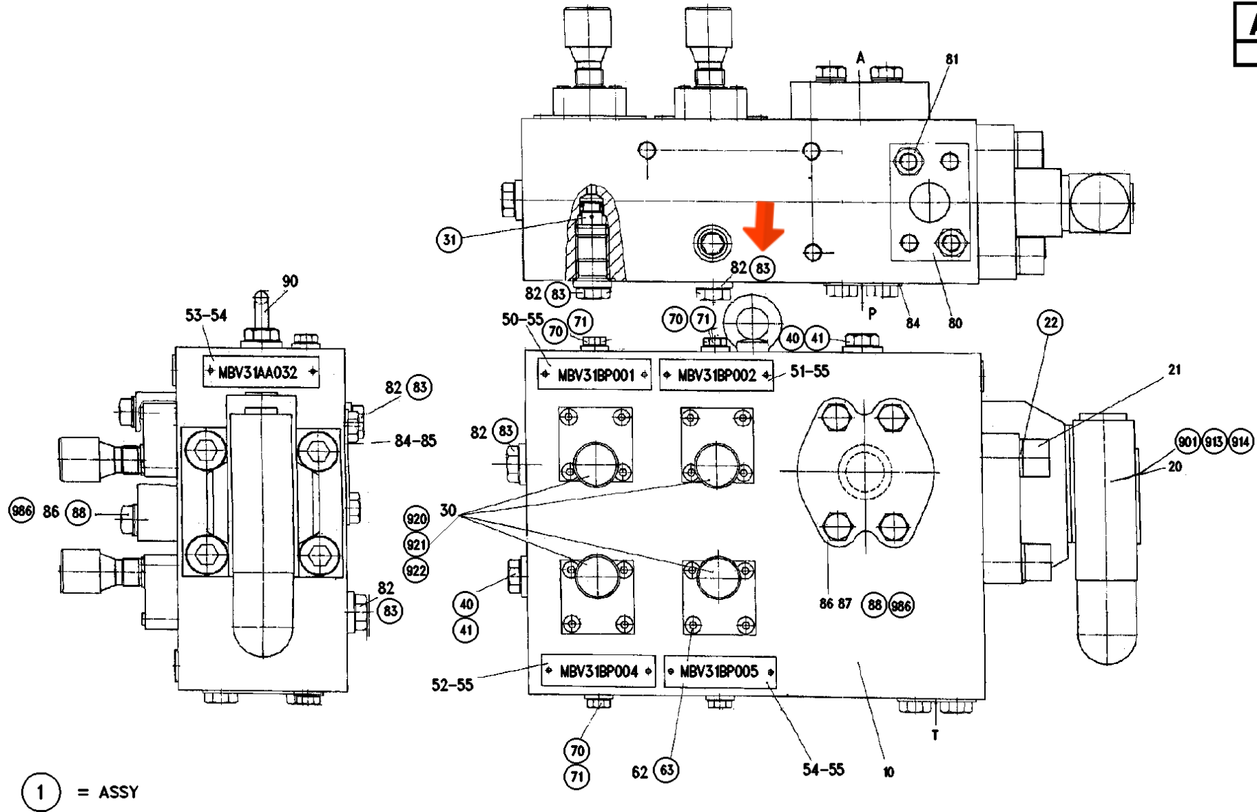
BLOCCO DI CONTROLLO OLIO DI SOLLEVAMENTO LIFTING OIL CONTROL BLOCK
