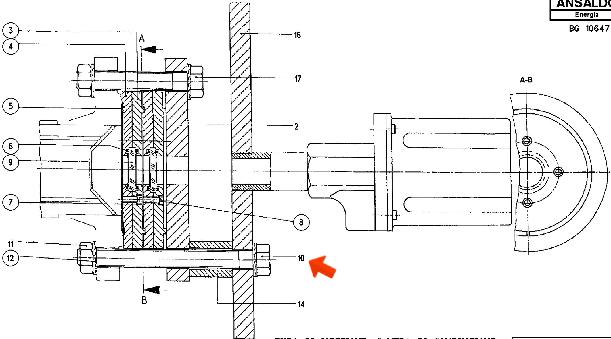
TUBO DI ISPEZIONE, CAMERA DI COMBUSTIONE INSPECTION TUBE AT COMBUSTION CHAMBER
