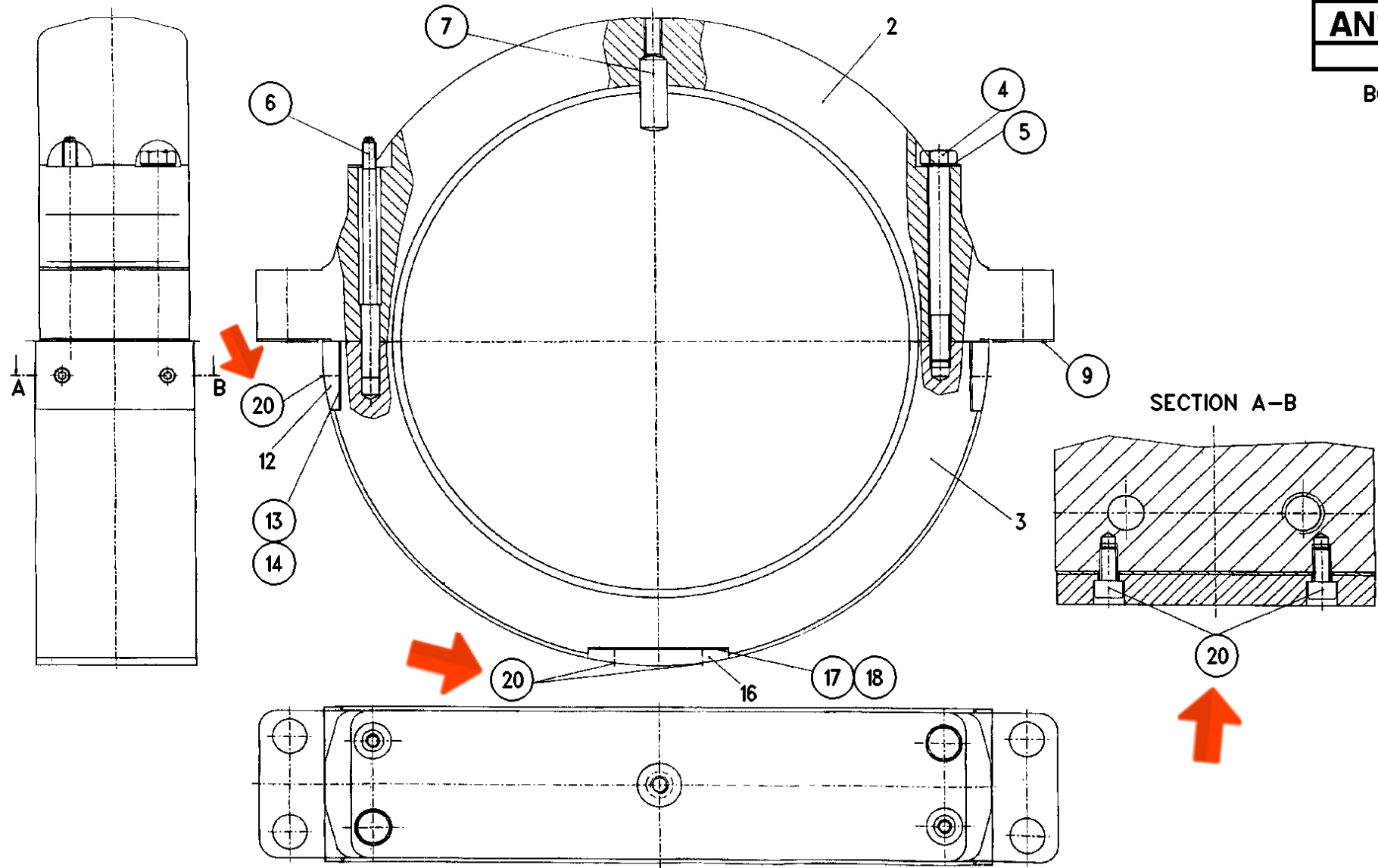
ANELLO ALLOGGIAMENTO CUSCINETTO ADJUST RING
