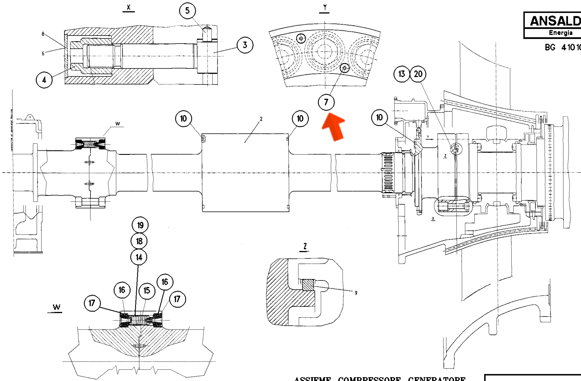
ASSIEME COMPRESSORE GENERATORE COMPRESSOR GENERATOR ASSEMBLY
