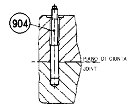
SECTION B-B SEZIONE B-B
