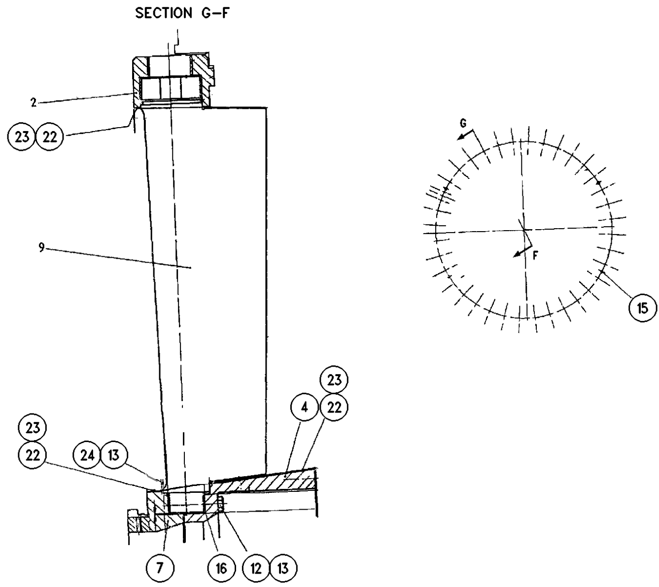
ANELLO PALE FISSE COMPR. STATORE 0 0TH COMPRESSOR STATOR BLADE RING
