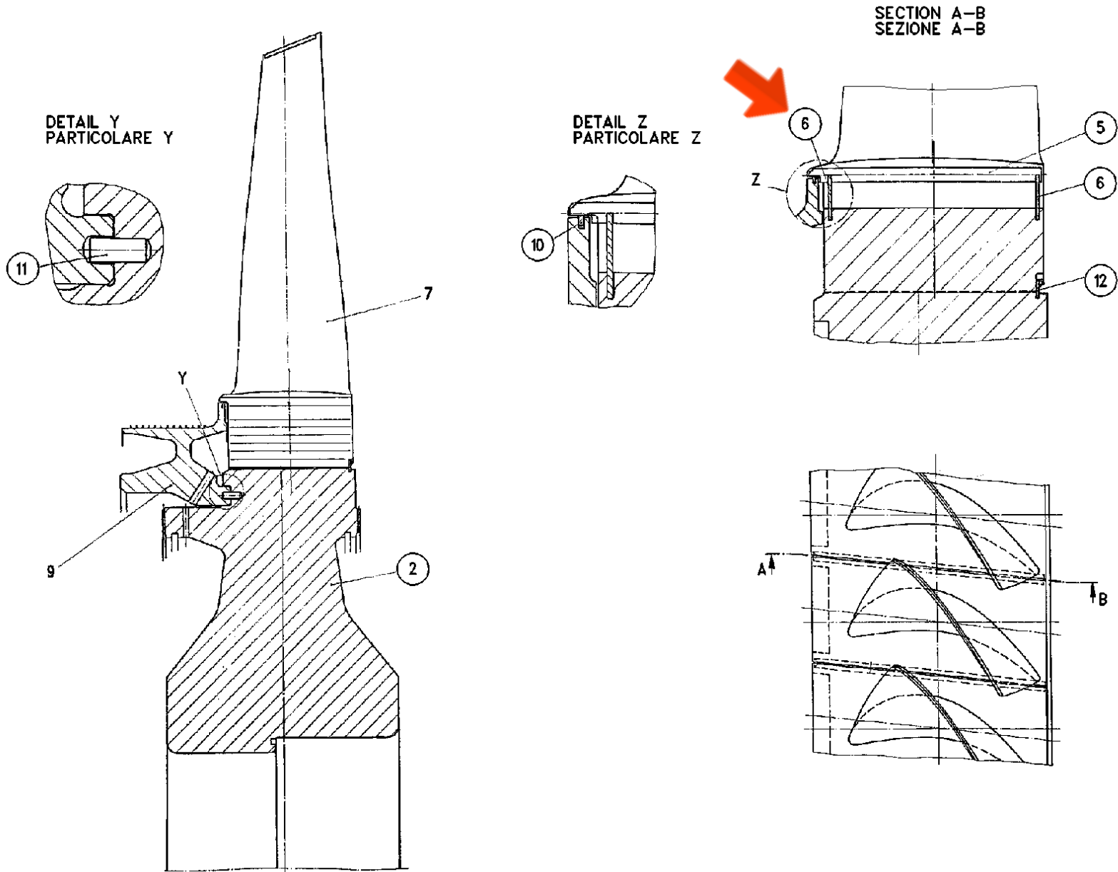
DISCO PALETTATO STADIO 4 BLADE WHEEL 4, TURBINE
